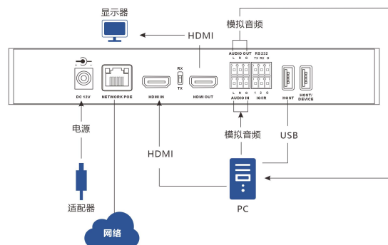
SP3500 输入模式
