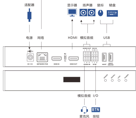
SP3500 输出模式
