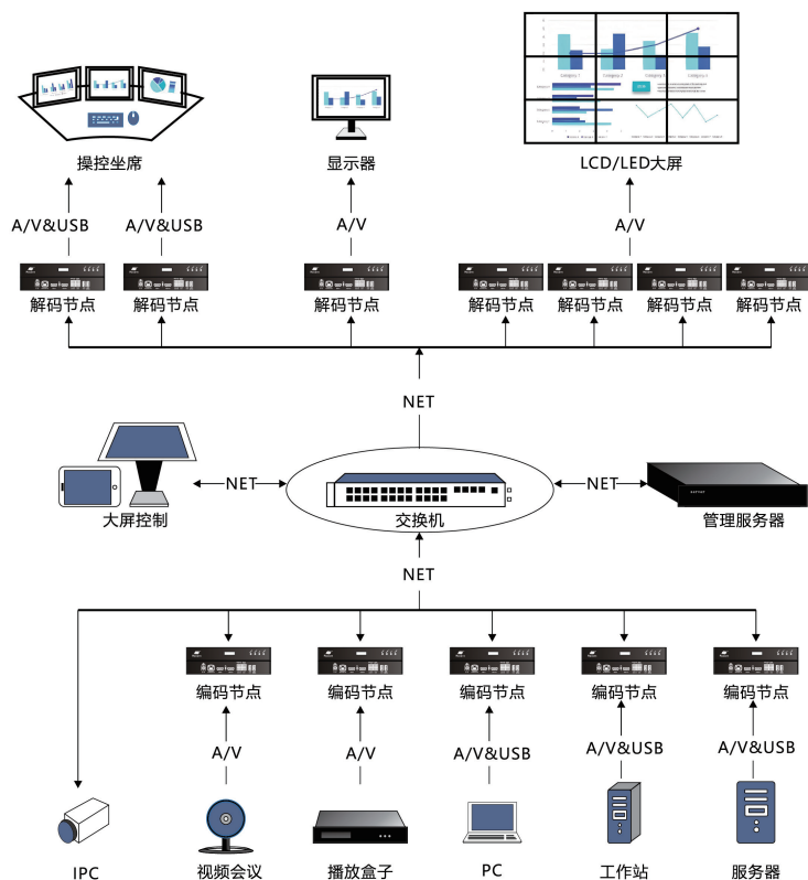
SP3500 输入模式
